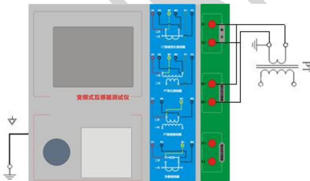
图 2.7 PT 直阻、励磁试验接线方式
