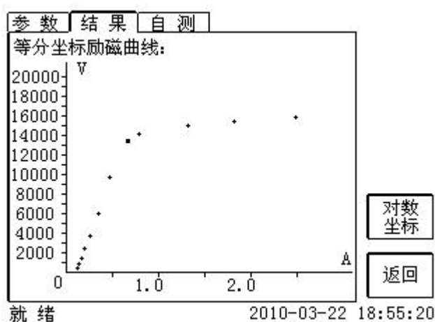
图 2.19 励磁曲线界面
